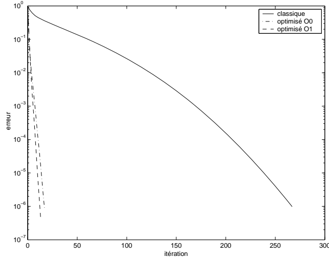
FIG. 1. L'erreur en fonction du nombre d'itérations. The error as a function of the number of iterations
