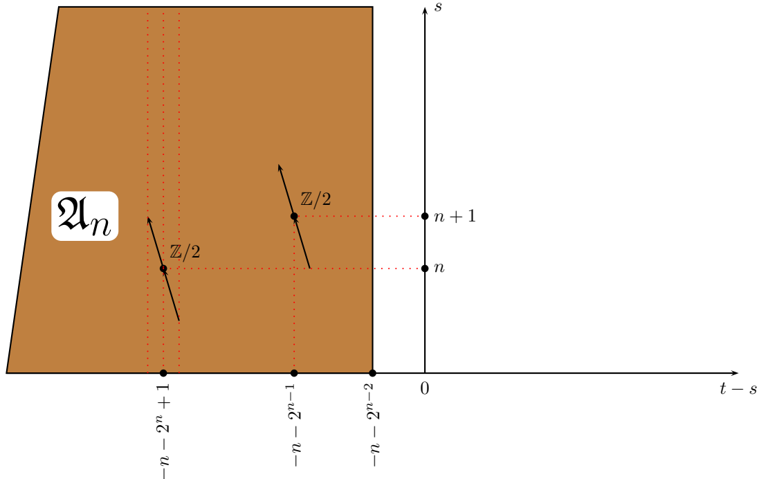
FIG. 1 – \mathrm{Ext}_{\mathcal{A}}^{s,t}(\mathbb{Z}/2, L'_n) , n \geq 2
