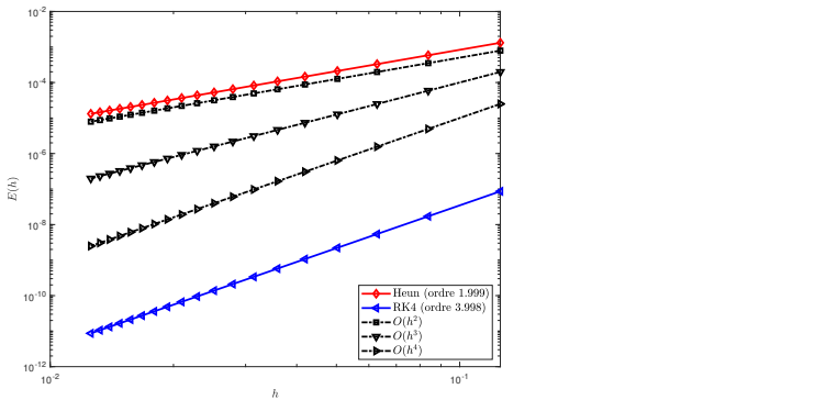
Figure: Méthode RK4 : vérification numérique de l'ordre
