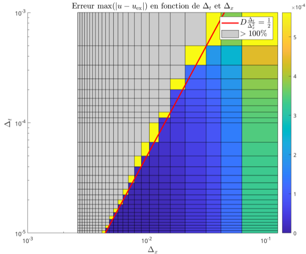
Figure: Equation de la chaleur 1D avec solution exacte. Condition de CFL \Delta_x \leq \sqrt{2 D \Delta_t}
