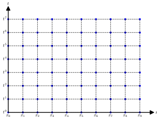
Figure: Grille espace-temps avec N_t = 7 et N_x = 9 .
