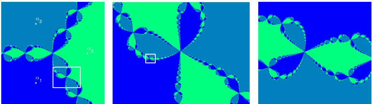
Figure 2.24: Méthode de Newton, système (2.34), zooms sur les bassins d'attraction
