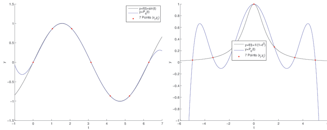
Figure 4.3: Polynômes d'interpolation de lagrange avec n = 6 (7 points) uniformément répartis. À gauche pour la fonction f : t \rightarrow \sin(t) avec x_0 = 0 , x_6 = 2\pi et à droite pour la fonction f : t \rightarrow 1/(1+t^2) avec x_0 = -5 , x_6 = 5 .
