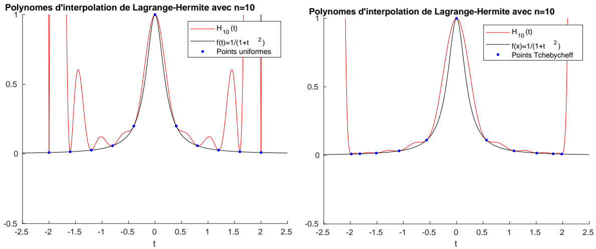
Figure 4.10: Polynôme d'interpolation de Lagrange-Hermite avec n = 10 (11 points) pour la fonction f : x \rightarrow 1/(1 + 25x^2) . A gauche avec des points uniformément répartis et à droite avec des points de Tchebychev
