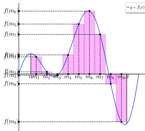
Figure 5.6: Formule composite des points milieux : \int_a^b f(x) dx \approx h \sum_{j=1}^k f(m_j) (aire de la surface colorée)
