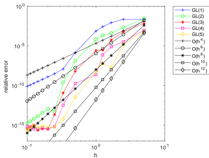
Figure 5.12: Erreur des méthodes de Gauss-Legendre composées pour le calcul de \int_{-5}^5 \frac{1}{1+x^2} dx , GL(n) correspondant à Q_{k,n}^{\text{comp}} et h = \frac{10}{k} .
