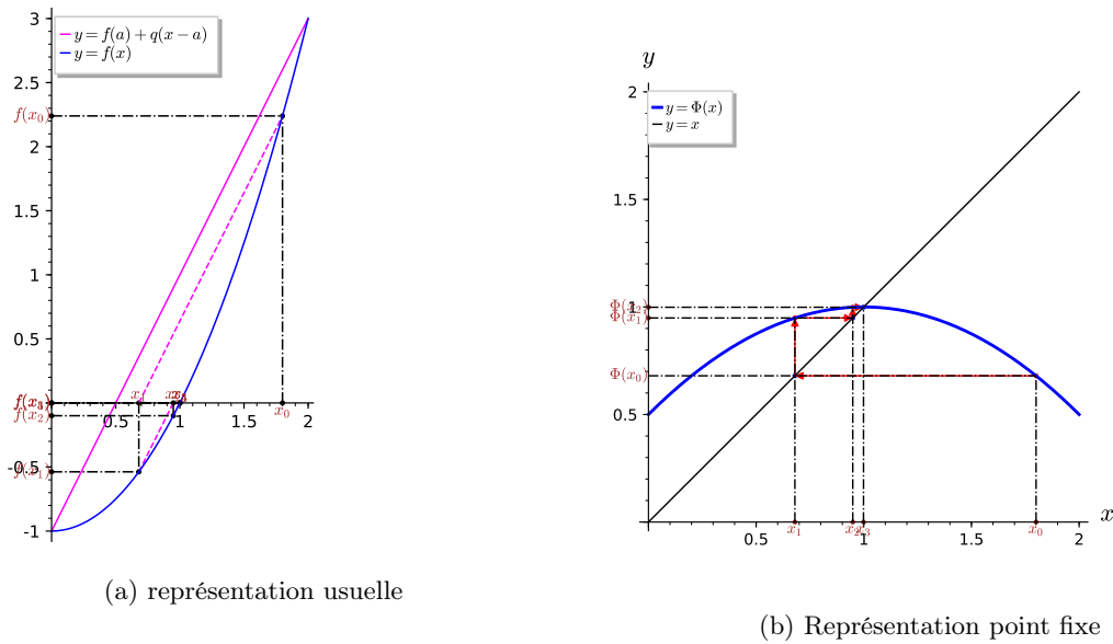
Figure 2.9: Exemple 1, méthode de la corde, \alpha = 1 , racine de f : x \mapsto x^2 - 1 avec a = 0.00 , b = 2.00 , x_0 = 1.80 ,
