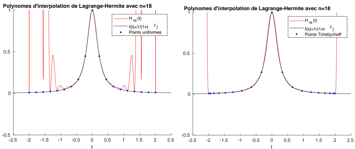
Figure 4.11: Polynôme d'interpolation de Lagrange-Hermite avec n = 18 (19 points) pour la fonction f : x \rightarrow 1/(1 + 25x^2) . A gauche avec des points uniformément répartis et à droite avec des points de Tchebychev
