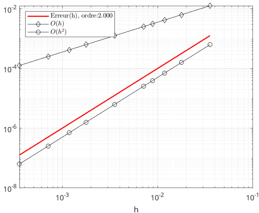
FIGURE 3 – Ordre du schéma représenté avec BVP0.order . Dans la légende, la valeur de l'ordre est déterminée numériquement.
