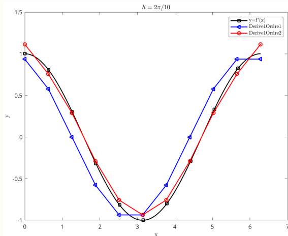
Figure: Représentation des dérivées numériques avec f(x) = \sin(x) , a = 0 , b = 2\pi . À gauche h = \frac{2\pi}{10} , à droite h = \frac{2\pi}{100} .
