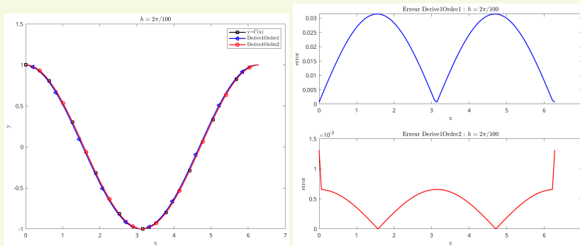
Figure: Avec f(x) = \sin(x) , a = 0 , b = 2\pi , N = 100 , à gauche, les différentes dérivées, à droite les erreurs commises par les deux fonctions.
