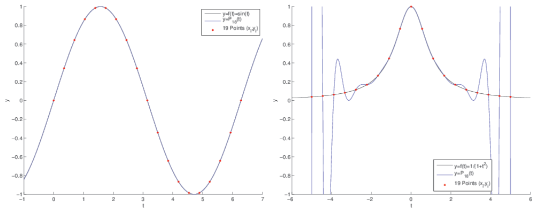
Figure 4.5: Polynômes d'interpolation de lagrange avec n = 18 (19 points) uniformément répartis. A gauche pour la fonction f : x \rightarrow \sin(x) avec x_0 = 0 , x_{18} = 2\pi et à droite pour la fonction f : x \rightarrow 1/(1 + x^2) avec x_0 = -5 , x_{18} = 5 .
