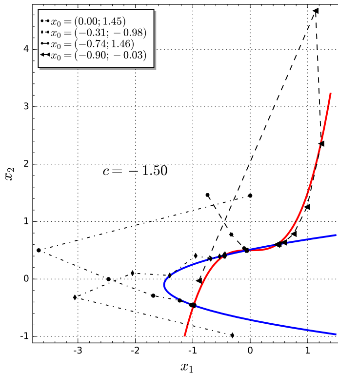
Figure 2.21: Représentation de 4 suites pour le système 2.33
