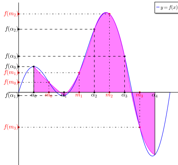
Figure 5.8: Formule composite de Simpson : \int_{\alpha}^{\beta} f(x)dx \approx \frac{h}{6} \left( 4 \sum_{j=1}^k f(m_j) + f(\alpha_0) + 2 \sum_{j=1}^{k-1} f(\alpha_j) + f(\alpha_k) \right) (aire de la surface colorée)
