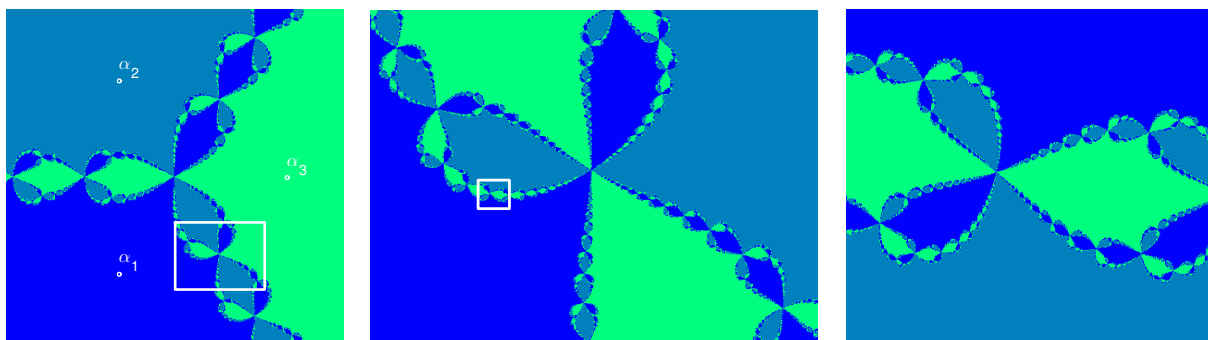
Figure 2.24: Méthode de Newton, système (2.34), zooms sur les bassins d'attraction
