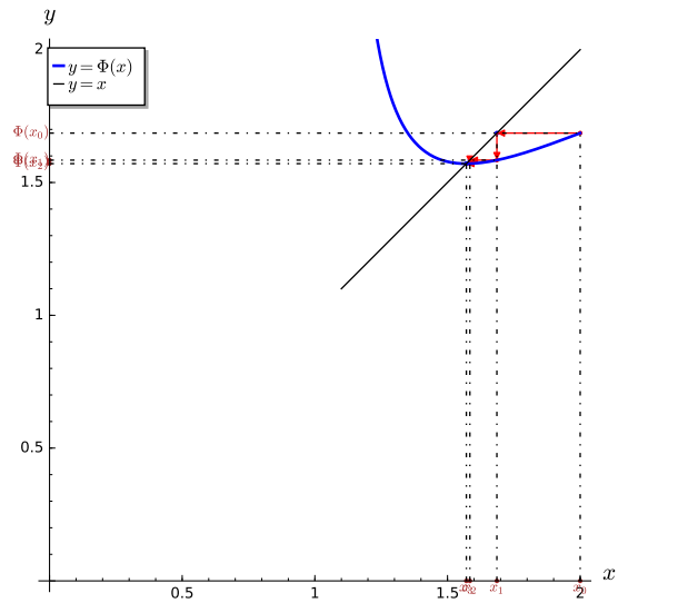
(b) Représentation point fixe, \Phi : x \mapsto \frac{x^2 \cos(x)}{x^2 \sin(x) - 2x \cos(x)} + x
