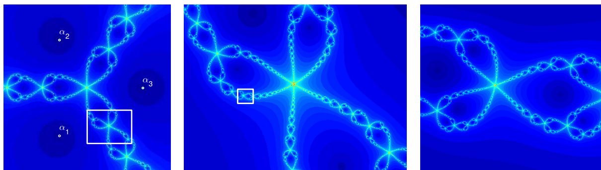
Figure 2.25: Méthode de Newton, système (2.34), zooms sur les nombres d'itérations
