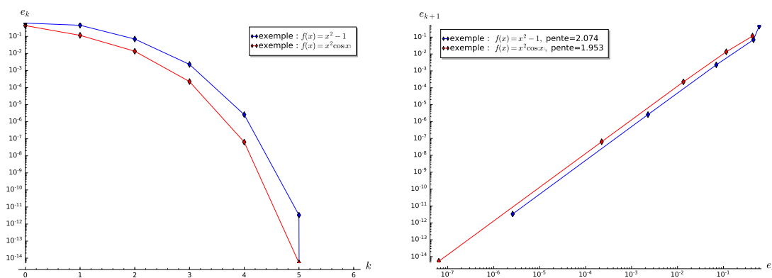
(a) Représentation de la convergence, e_k en fonction de k
