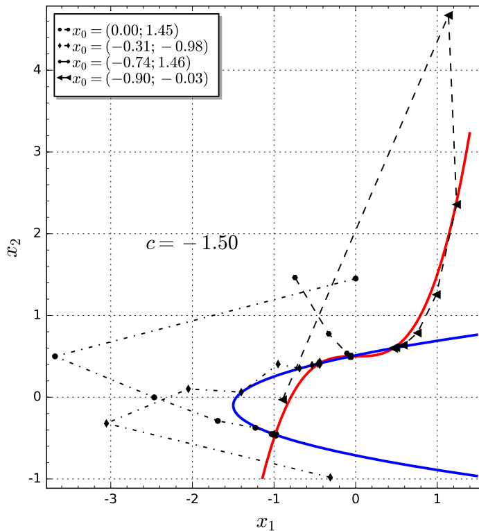
Figure 2.21: Représentation de 4 suites pour le système 2.33
