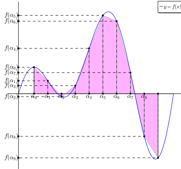
Figure 5.7: Formule composite des trapèzes : \int_a^b f(x)dx \approx \frac{h}{2} \left( f(\alpha_0) + 2 \sum_{j=1}^{k-1} f(\alpha_j) + f(\alpha_k) \right) (aire de la surface colorée)
