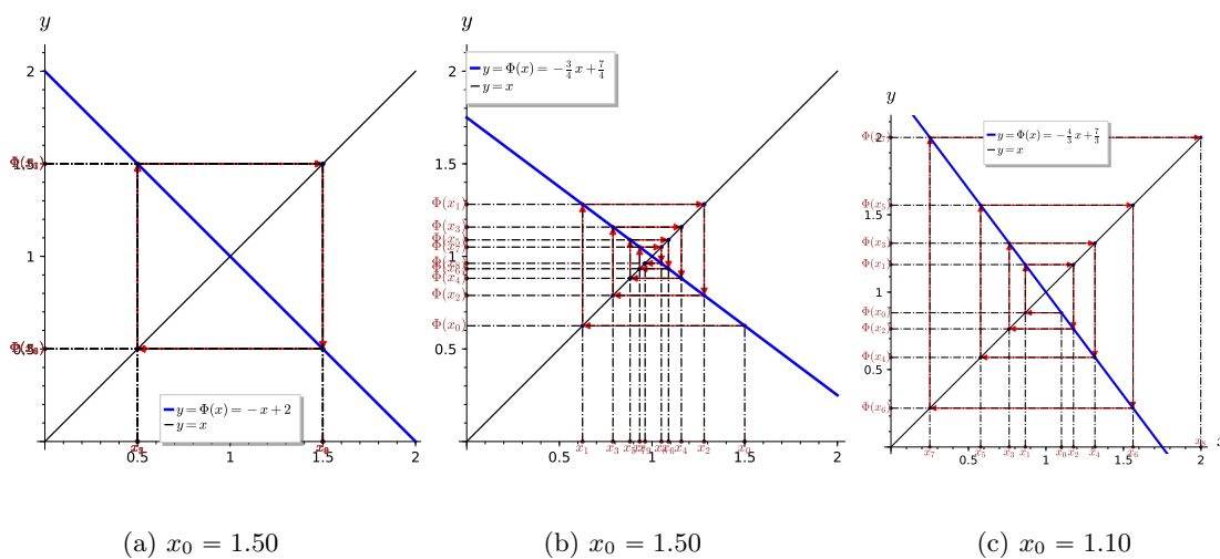
Figure 2.8: \alpha = 1 , point fixe de fonctions affines particulières
