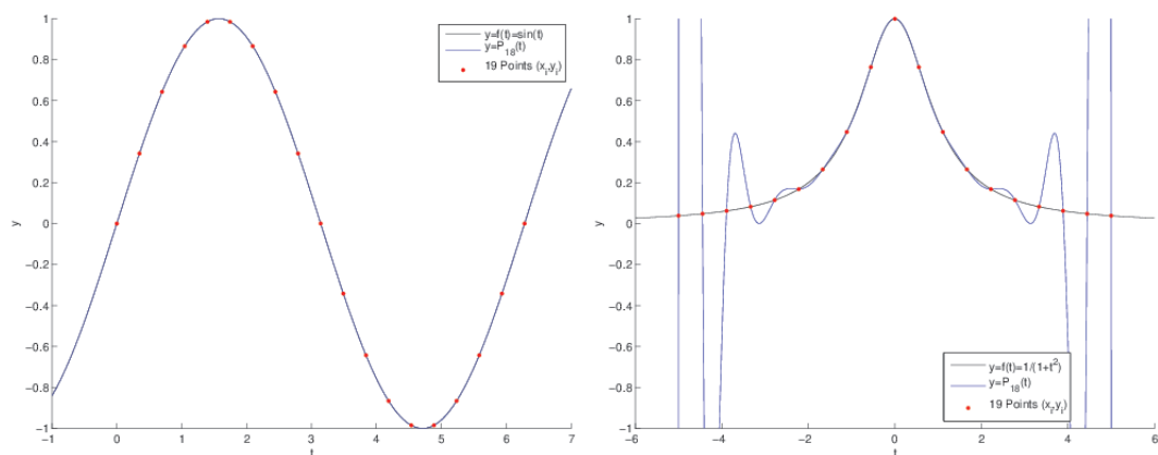
Figure 4.5: Polynômes d'interpolation de lagrange avec n = 18 (19 points) uniformément répartis. À gauche pour la fonction f : t \rightarrow \sin(t) avec x_0 = 0 , x_{18} = 2\pi et à droite pour la fonction f : t \rightarrow 1/(1+t^2) avec x_0 = -5 , x_{18} = 5 .
