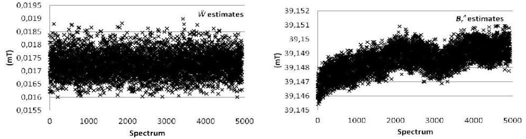
FIGURE 6.7 – Valeurs FWHM et \hat{B}_r estimées pour 5000 spectres RPE du même échantillon de TAM avec un rapport SNR de 7dB environ.
