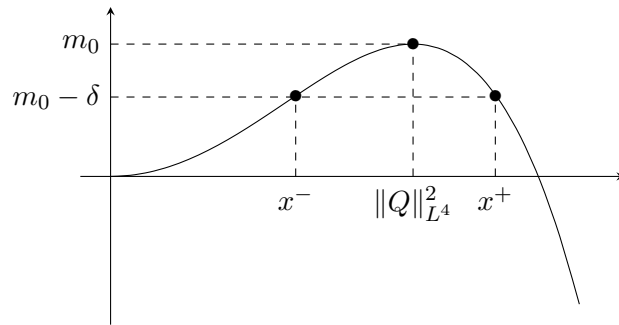
FIGURE 2.2 : Le graphe de \alpha .
