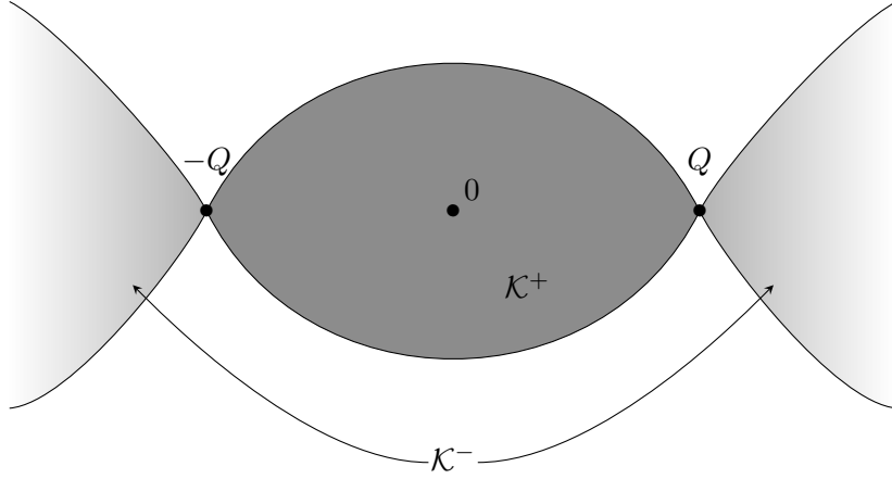
FIGURE 2.1 : Les ensembles \mathcal{K}^+ (en gris foncé) et \mathcal{K}^- (en dégradé).
